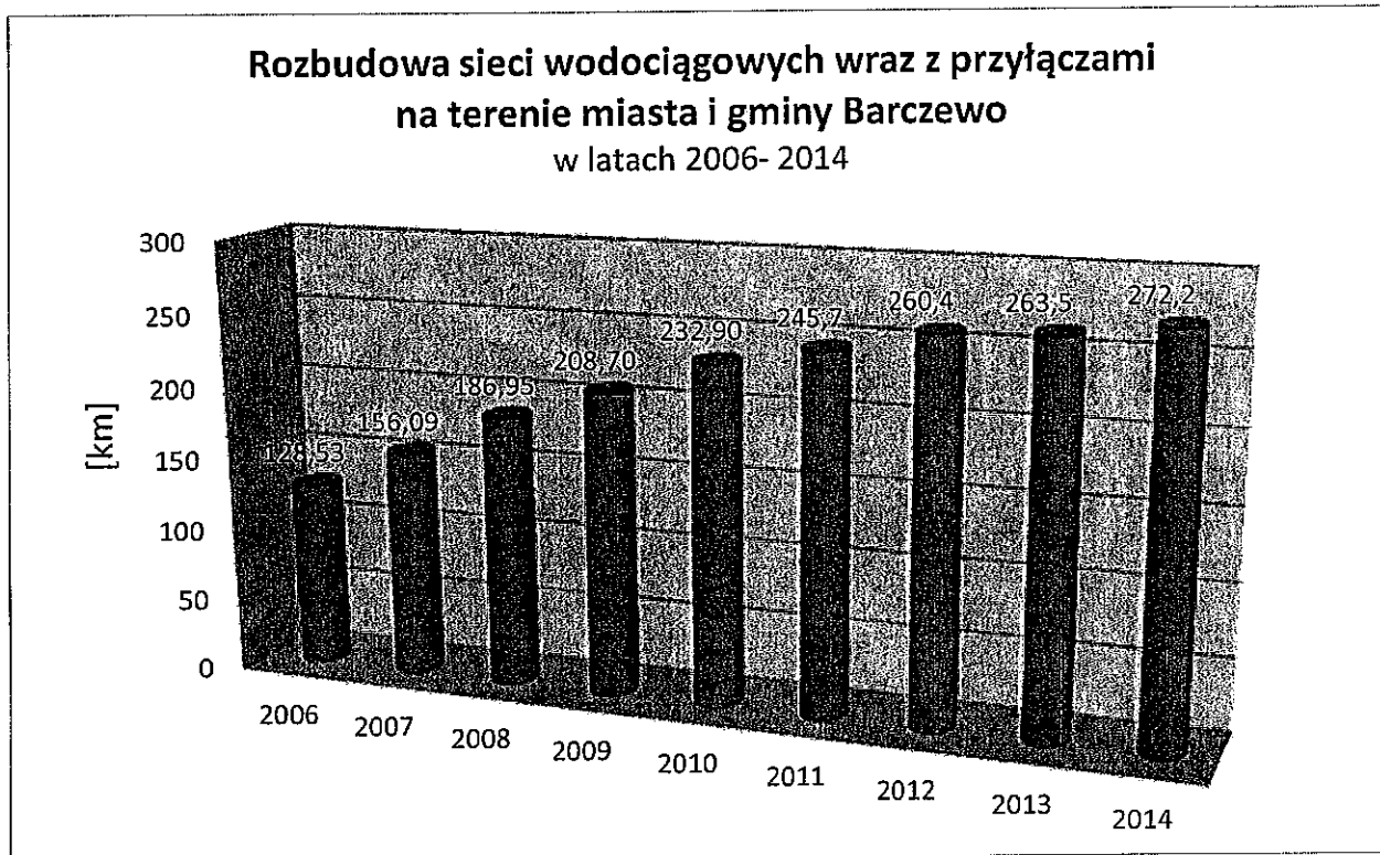
Rys. 4. Przyrost długości sieci wodociągowych na terenie miasta i gminy Barczewo w poszczególnych latach [km] wpływający na wartość podatku
