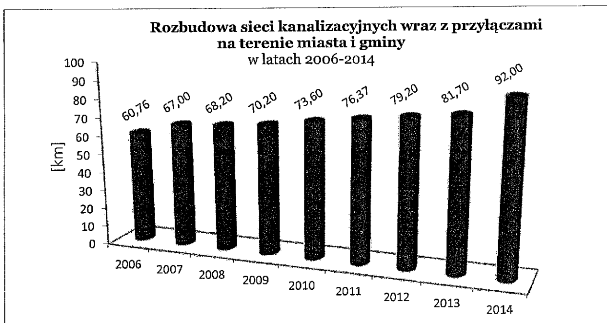
Rys. 5. Przyrost długości sieci kanalizacyjnych na terenie miasta i gminy Barczewo w poszczególnych latach [km] wpływający na wartość podatku
