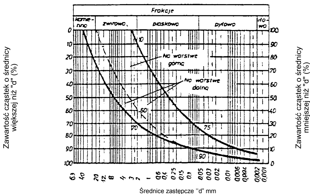
Rysunek 2. Obszar uziarnienia optymalnych mieszanek gliniasto-żwirowych
