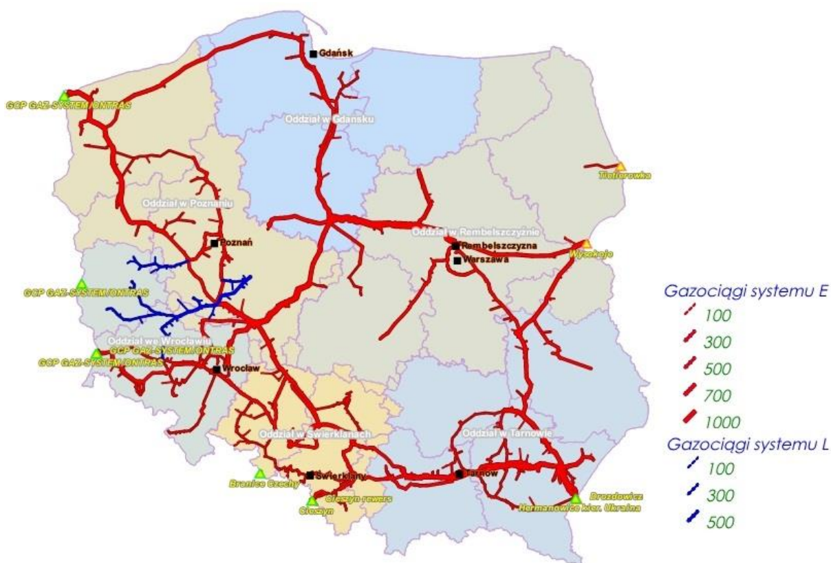
Rys. 27. Mapa systemu przesyłowego GAZ-SYSTEM S.A. źródło: www.gaz-system.p
