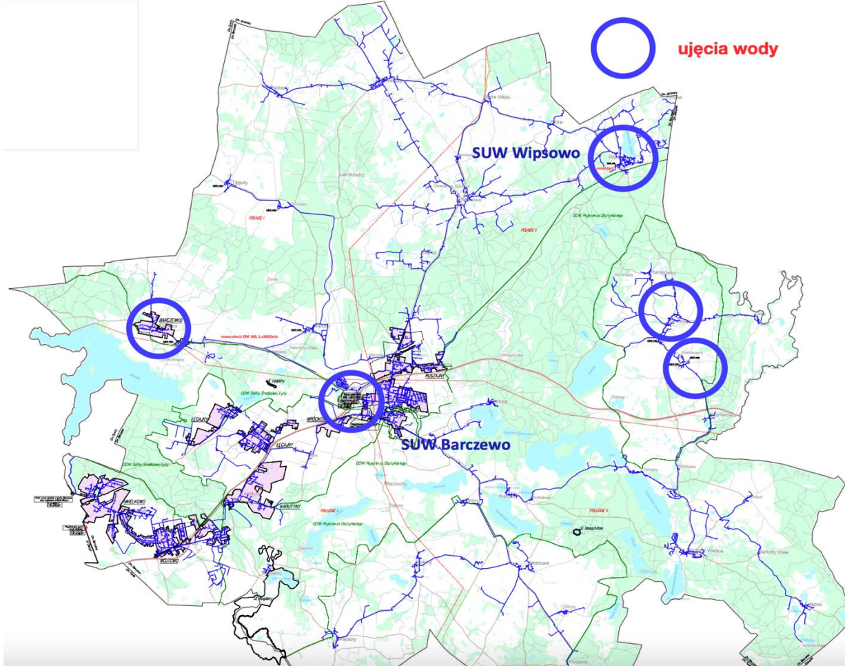
Rys. 1. Mapa Gminy Barczewo z lokalizacją sieci wodociągowej
